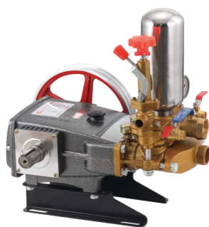
120型柱塞泵
